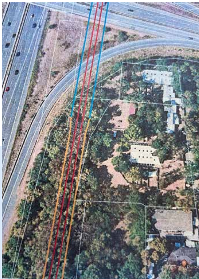
Geplante IC Trasse (rot) Trog (gelb) Tunnel (blau)
